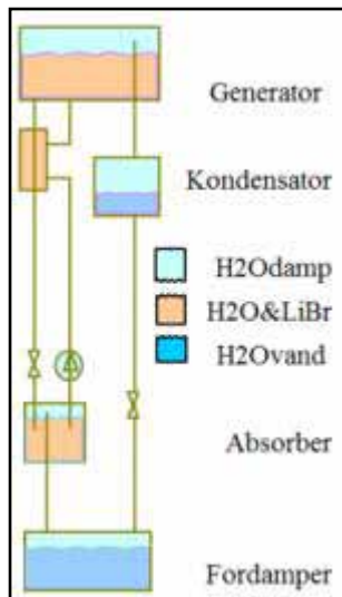
Principdiagram for en absorptionsvarmepumpe.
